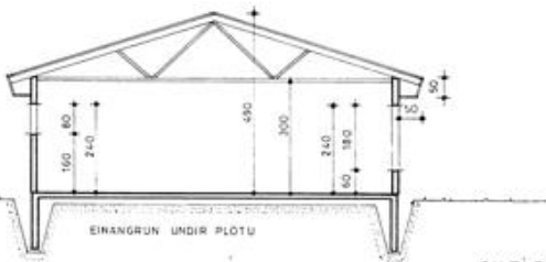
SNEIÐING A-A 1:100
