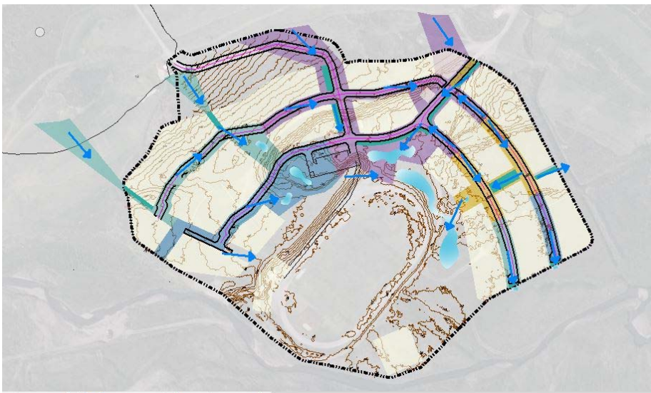
Mynd 6 Skýringarmynd fyrir leiðir ofanvatns og grófhönnun.
